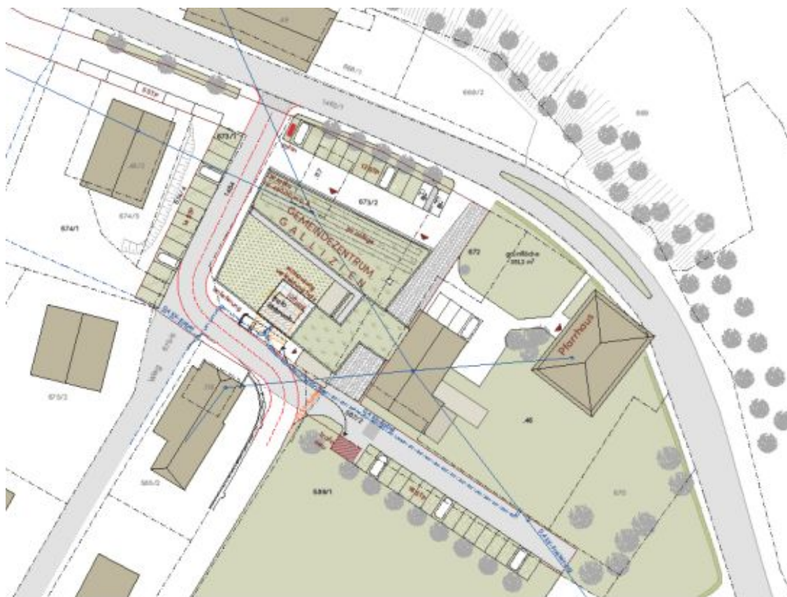
Abb. Lageplan (Quelle: MURERO BRESCIANO architektur ZT GmbH)
